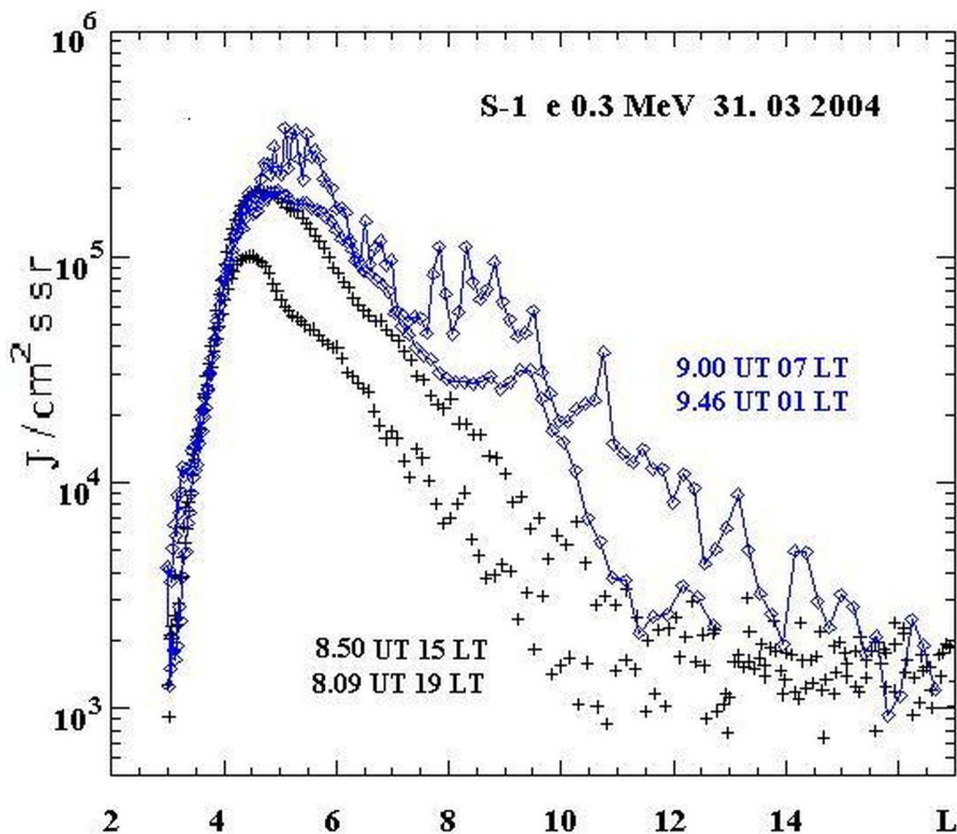
Рис 5б. Широтные профили, измеренные на S-1 31.03.2004 г. Времена пролетов обозначены.
