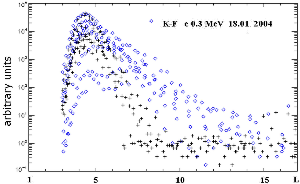
Рис 2. То же, что на рис 1а для интервала с повышенной суббуревой активностью.
