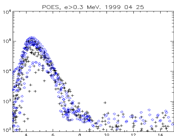
Рис 1. Примеры измерения радиальных профилей электронов, за несколько часов спокойной магнитной обстановки на спутниках К-Ф (а), S-1 (б) и POES-15 (в). Приведены все измерения без отбора, по четыре профиля за каждый облет Земли, как в северном так и в южном полушарии на восходящих и нисходящих орбитах. Ромбики (синие) — утренний сектор (00-12 LT), крестики (черные) -вечерний сектор (12-24 LT) .
