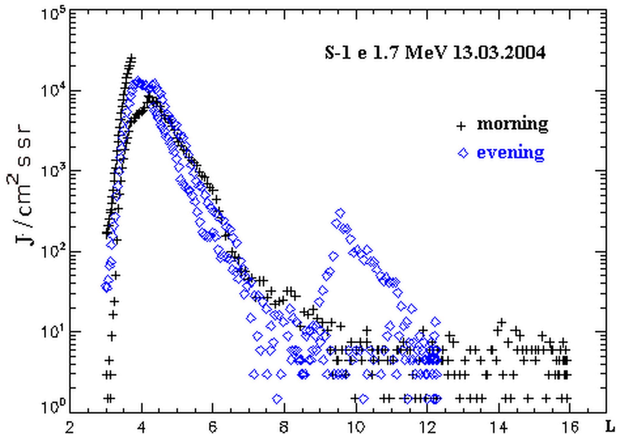
Рис 6 (б) . Широтные профили 13.03 2004.
